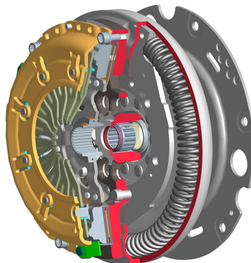
Fig. 2: A massa secundária é introduzida com um rolamento de agulhas no veio primário da caixa de velocidades
