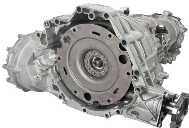
Fig. 1: Caixa de velocidades com o módulo da embraiagem montado
