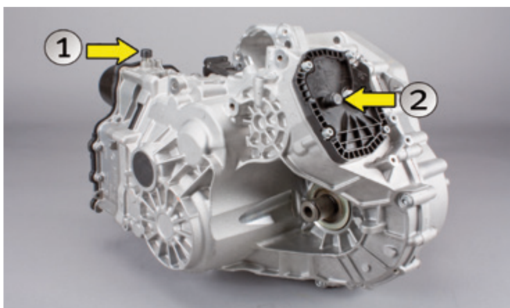
Fig. 1: Caixa de velocidades automática com tampas de purga para a mecatrónica (1) e a caixa de velocidades (2)
