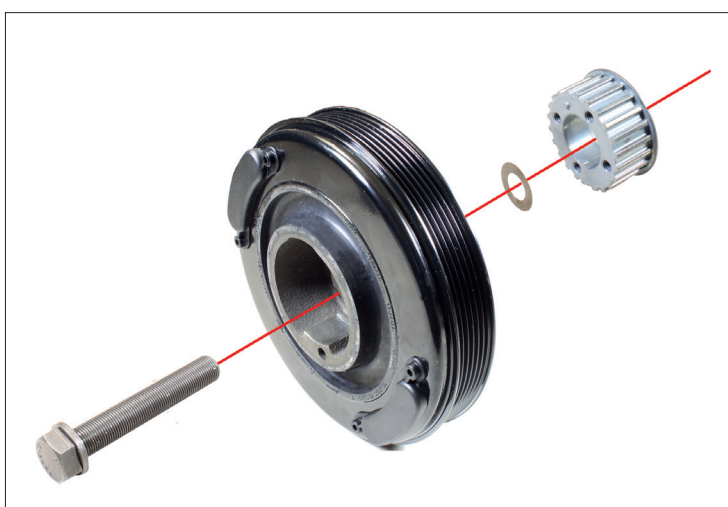
Fig. 1: Polia damper da cambota com parafuso central da mesma e anilha com recobrimento de diamante
